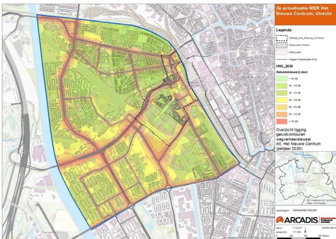
Figuur 11 Berekende geluidcontouren plansituatie “Beurskwartier en Lombokplein”, peiljaar 2030
