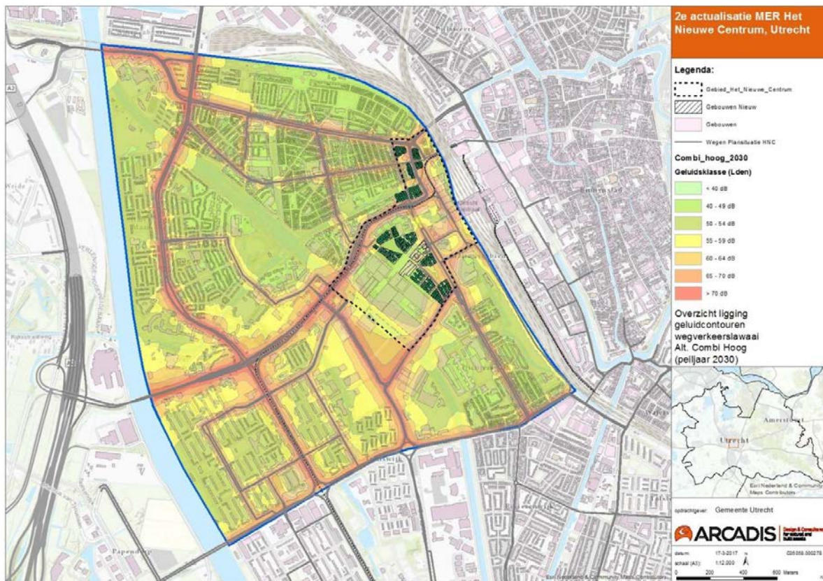
Figuur 12 Berekende geluidcontouren “Combi Hoog”, peiljaar 2030
